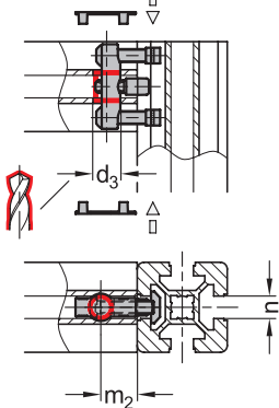
Montáž a obrábění profilu
